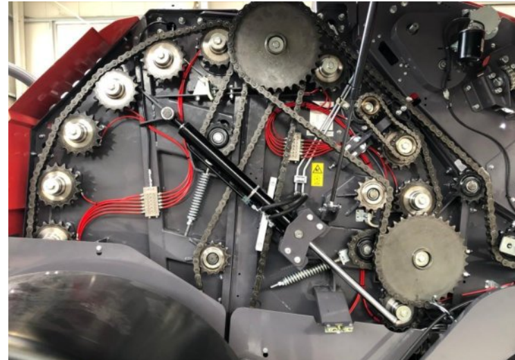
Automatische Kettenspanner
