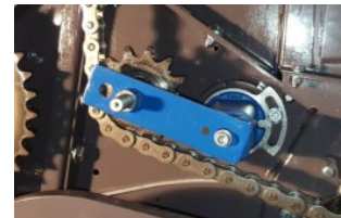
Automatische Kettenspanner
